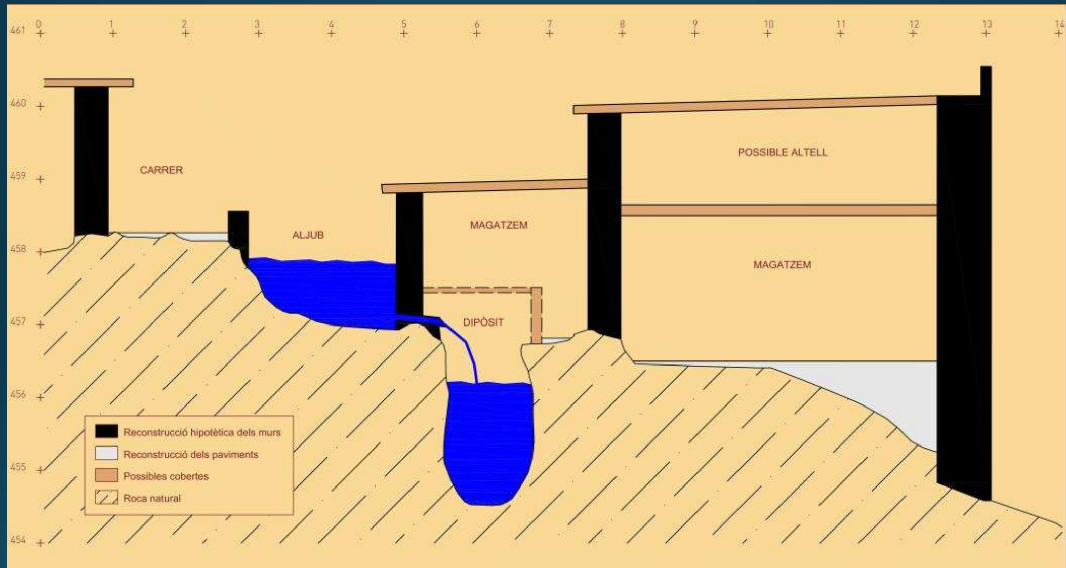
Secció del sistema de recollida d'aigua, amb la recreació hipotètica de l'edifici. Segons J.Chorén.
