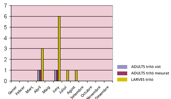
Nombre d'exemplars de tritó detectats durant l'any 2010
