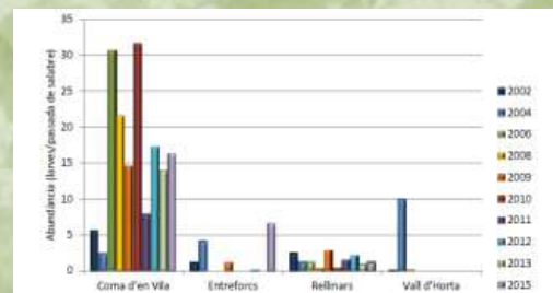
Figura 5.6. Evolució de l'abundància màxima de larves de granota verda (larves/passa de salobre) en les diferents estacions de seguiment.
