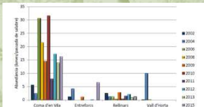
Figura 6.6. Evolució de l'abundància màxima de larves de granota verda (larves/passada de salatre) en les diferents estacions de seguiment.
