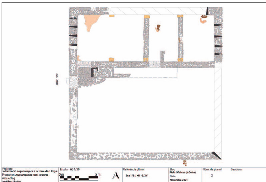
Figura 4. Planta general de la fase baixmedieval de la torre d'en Pega
