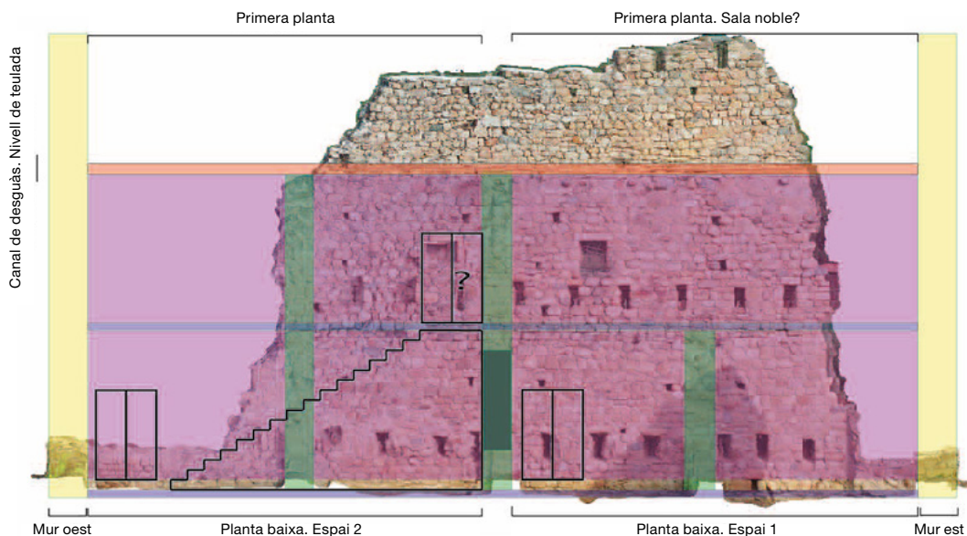
Figura 2. Vista esquemàtica del mur nord
