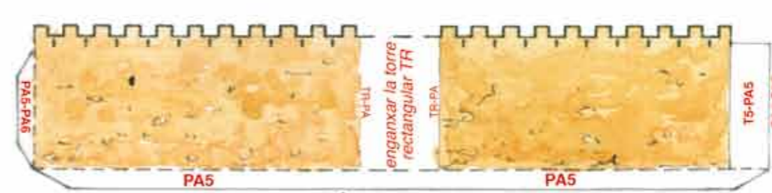
Murs recinte pati d'armes
